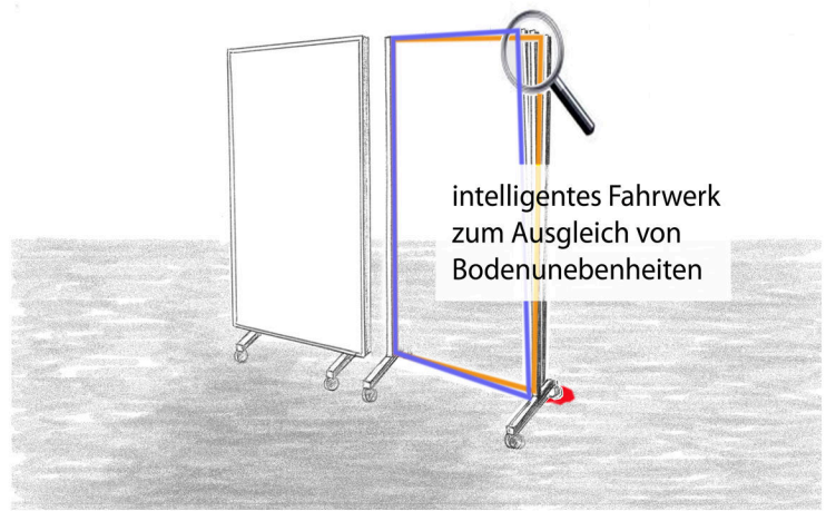
Justagemöglichkeit zur Angleichung der Höhe bei nebeneinander stehenden Absorbern
